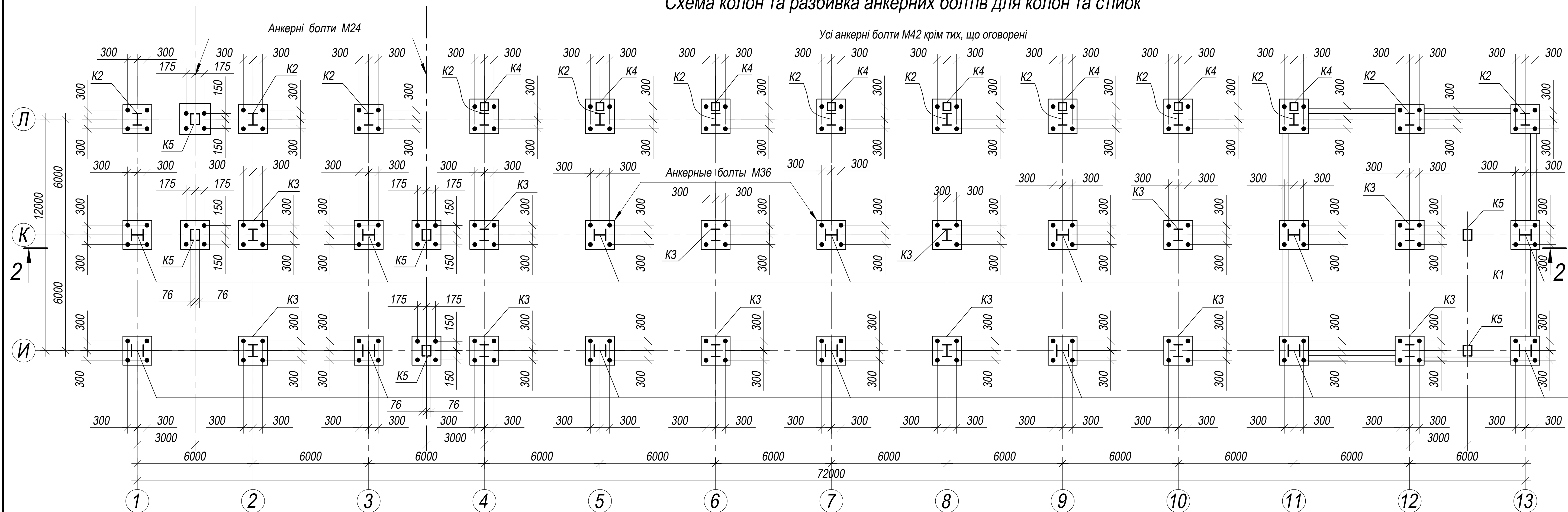
Схема колон та розбивка анкерних болтів для колон та стійок
