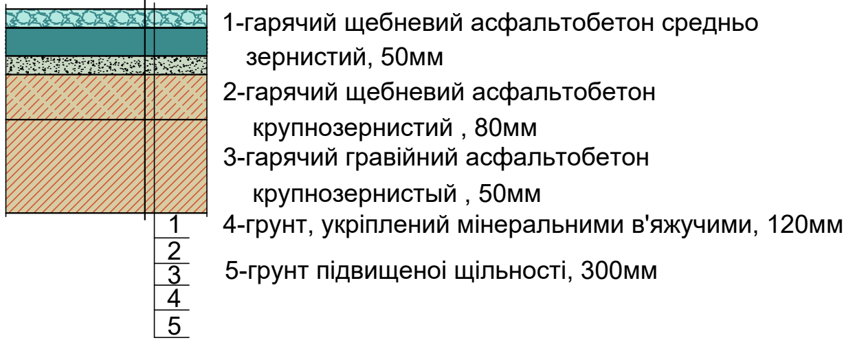
Переріз проїзду
