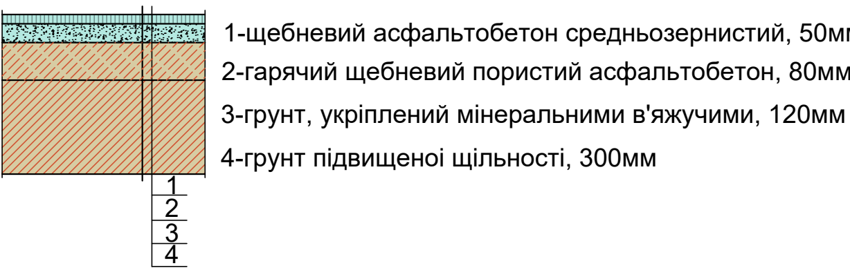
Переріз тротуару
