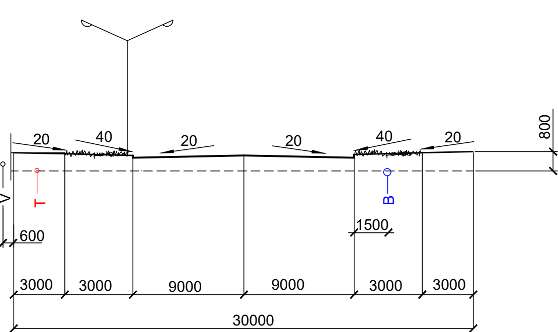
Розріз 2-2
