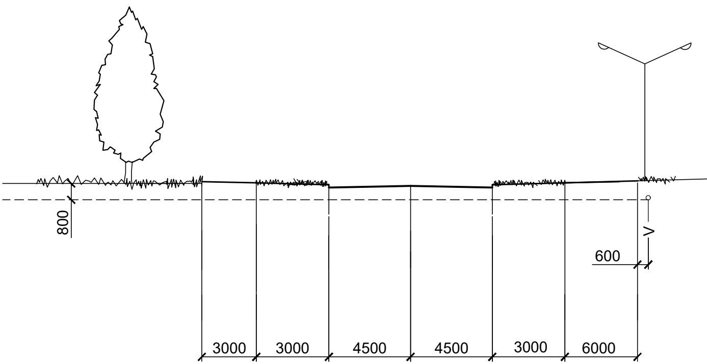
Розріз 1-1
