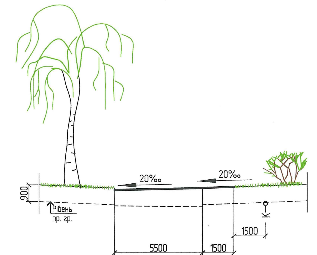
Розріз 2-2
