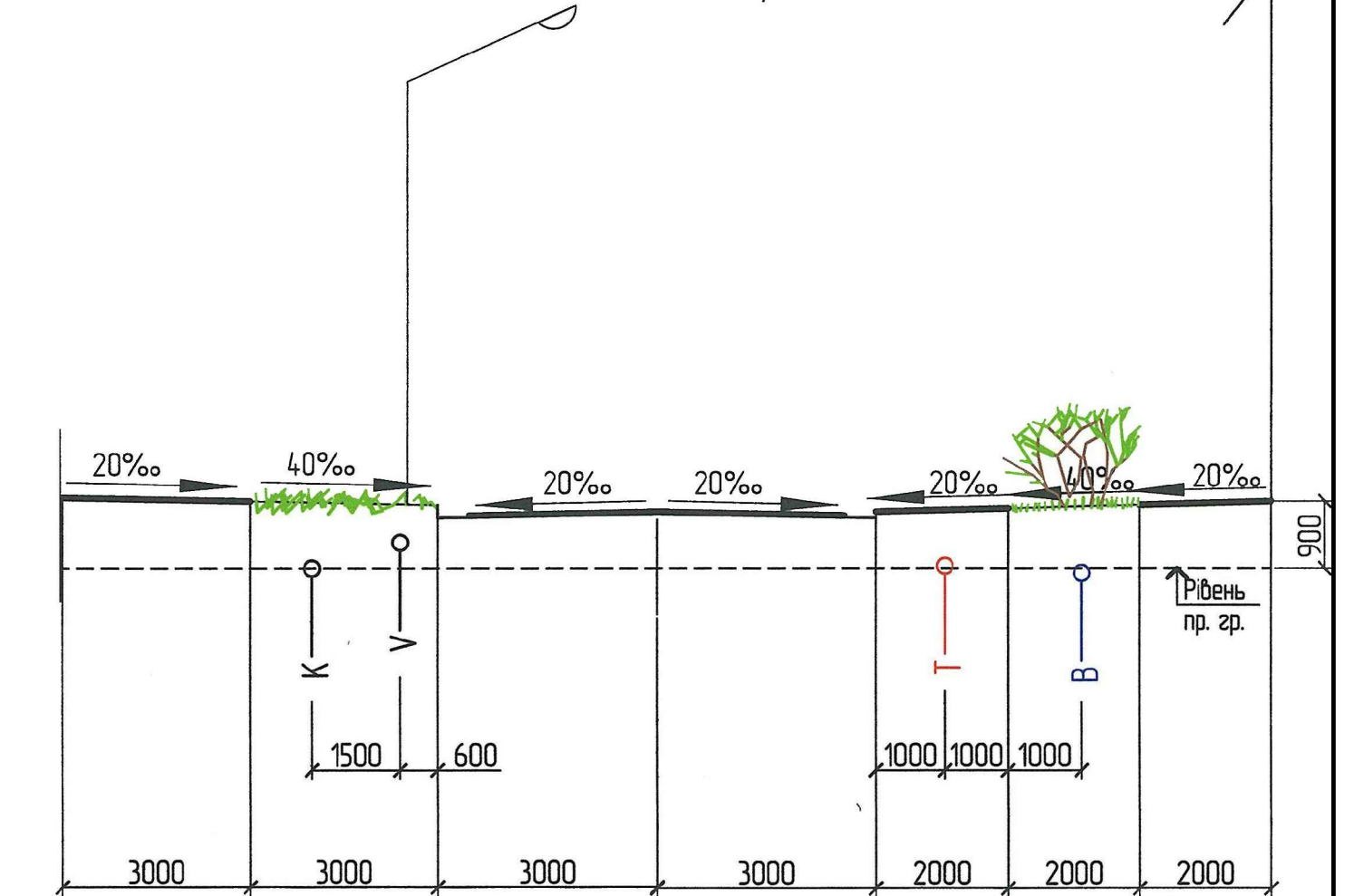
Розріз 1-1
